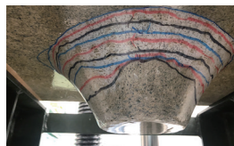
▲押し抜試験状況
