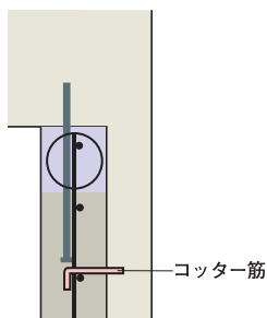
増厚壁の配筋詳細図
