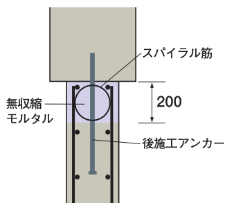
増設壁の配筋詳細図
