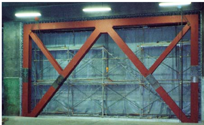
鉄骨ブレース工法(在来工法)
