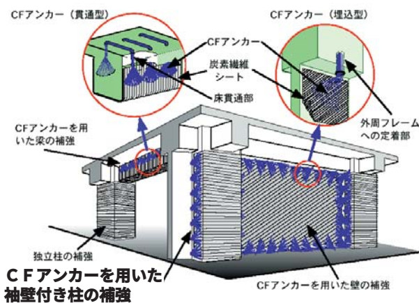
④ SR-CF工法による建物の耐震補強
