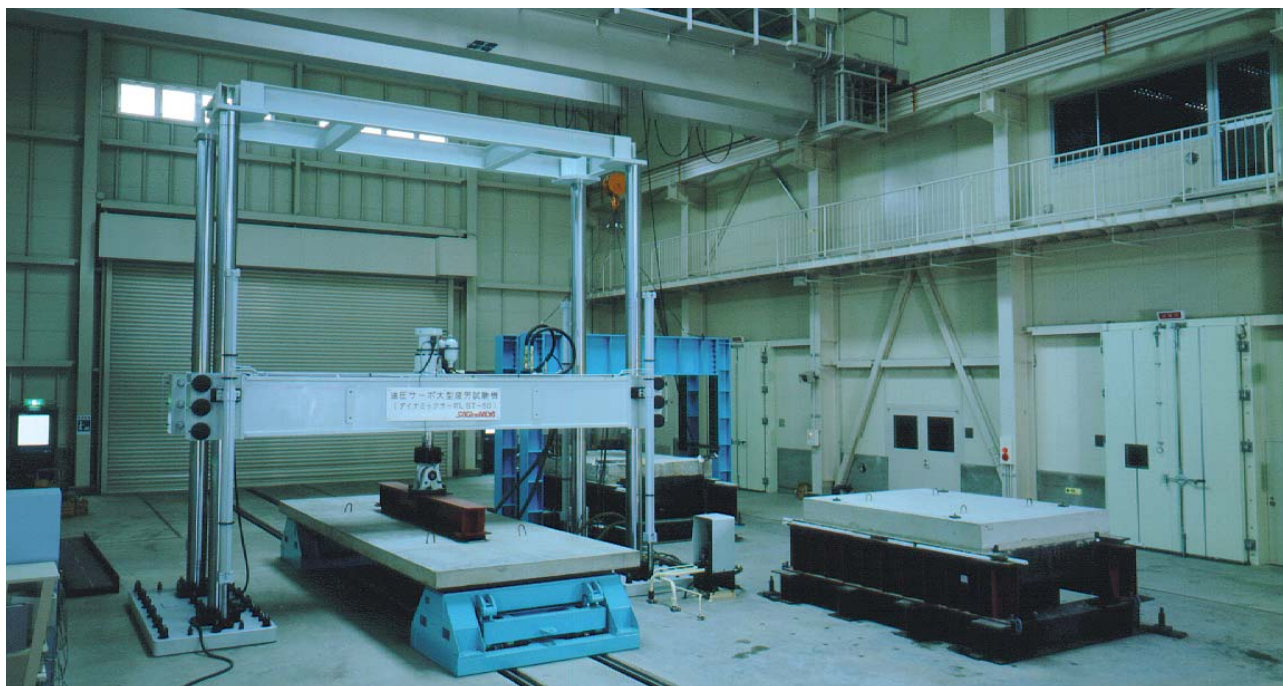
500kN構造物疲労試験機が設置された大型実験室
